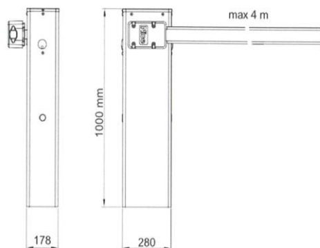
Габариты
